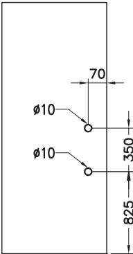
XL - C 3003A (D Type Handle - 450 x 25 mm)
