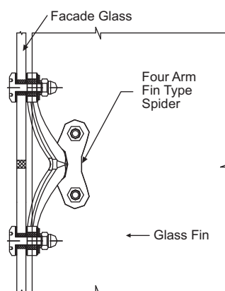
Elevation
